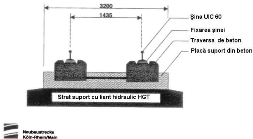
Figura 3. Secțiune tip prin calea durabilă cu traverse bi-bloc
