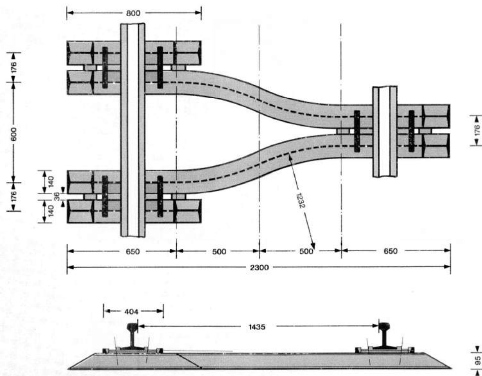
Figura 1. Forma și dimensiunile principale ale traversei metalice Y
